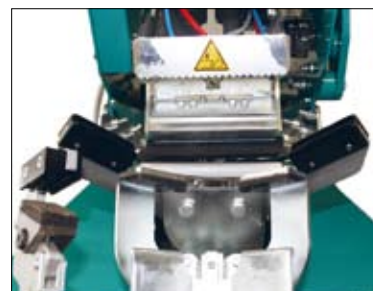
Benklemmen fikserer bagbenene, som er løsnet fra skindet på Combi Cut.
