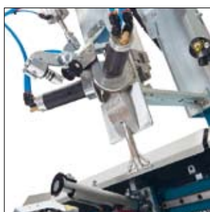
Den todelte slaglængde på bugløsneren gør maskinen endnu hurtigere.
